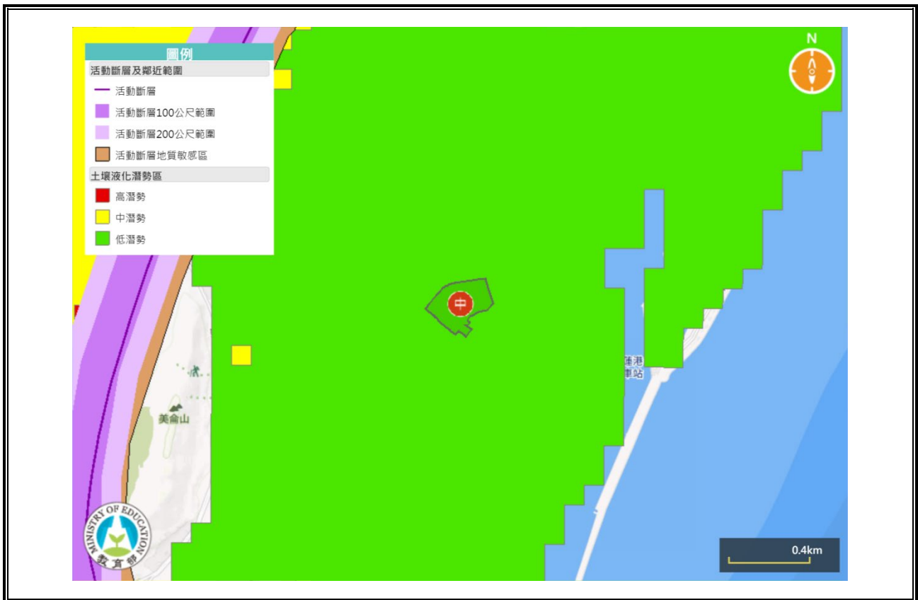
圖 2.4.1 地震災害潛勢圖 (瀏覽日期：113 年 05 月 24 日)
